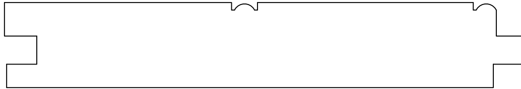
PA5375 7/8" x 5-3/8"
